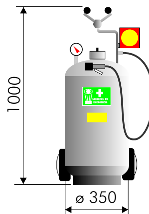
ARTICULO 6050 LAVAJOS DIMENSIONES EN mm
