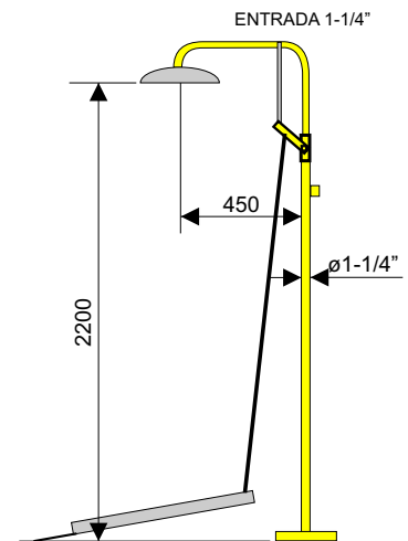
ARTICULO 6016 DUCHA CON LAVAOJOS DIMENSIONES EN mm
