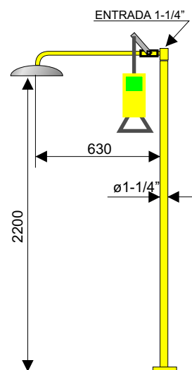
ARTICULO 6015 DUCHA DE EMERGENCIA DIMENSIONES EN mm
